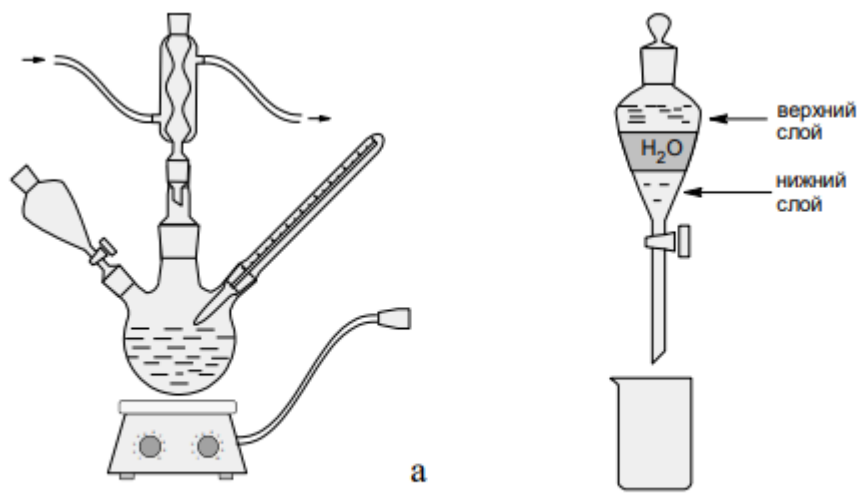
Рис. 1. Схема прибора для нитрования бензола
